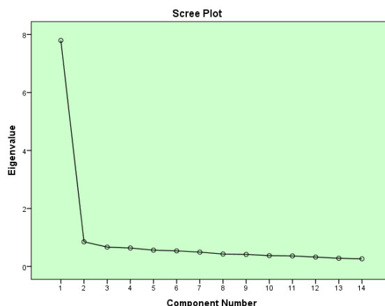
نمودار ۲: آزمون اسکری مربوط به عوامل بازدارنده مطالعه
