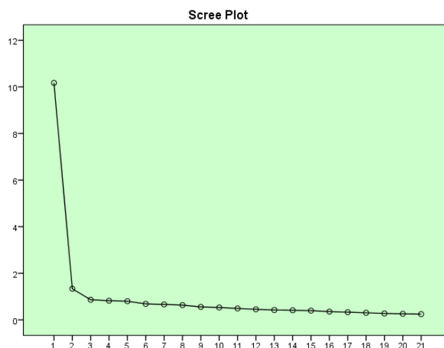
نمودار ۱: آزمون اسکری مربوط به عوامل ترغیب کننده مطالعه Chart 1: Scree Test for Supportive Factors of Studing
